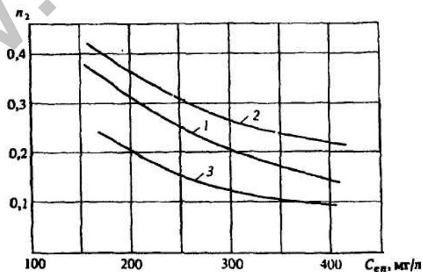
Черт. 2. Зависимость показателя степени n_2 от исходной концентрации взвешенных веществ в городских сточных водах при эффекте отстаивания 1 - \Theta = 50\% ; 2 - \Theta = 60\% ; 3 - \Theta = 70\%
